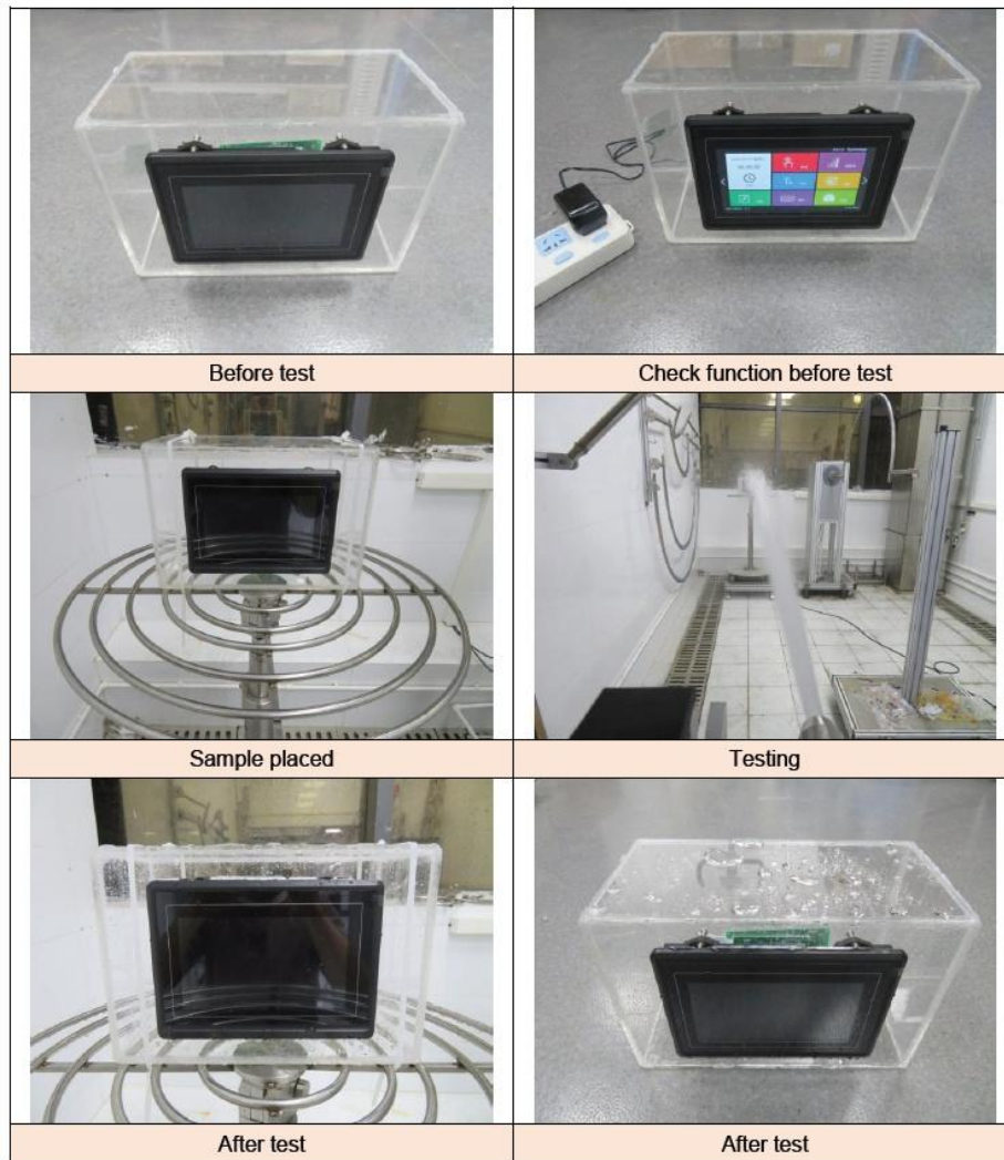
图 5-7 防水测试图
