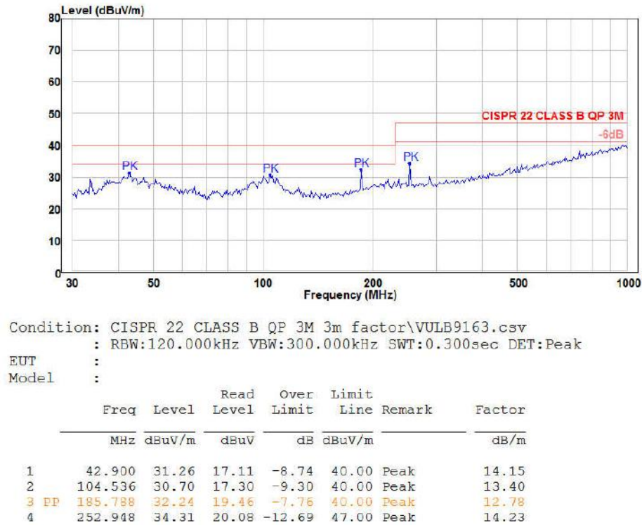
图 5-6 RE 测试垂直方向
