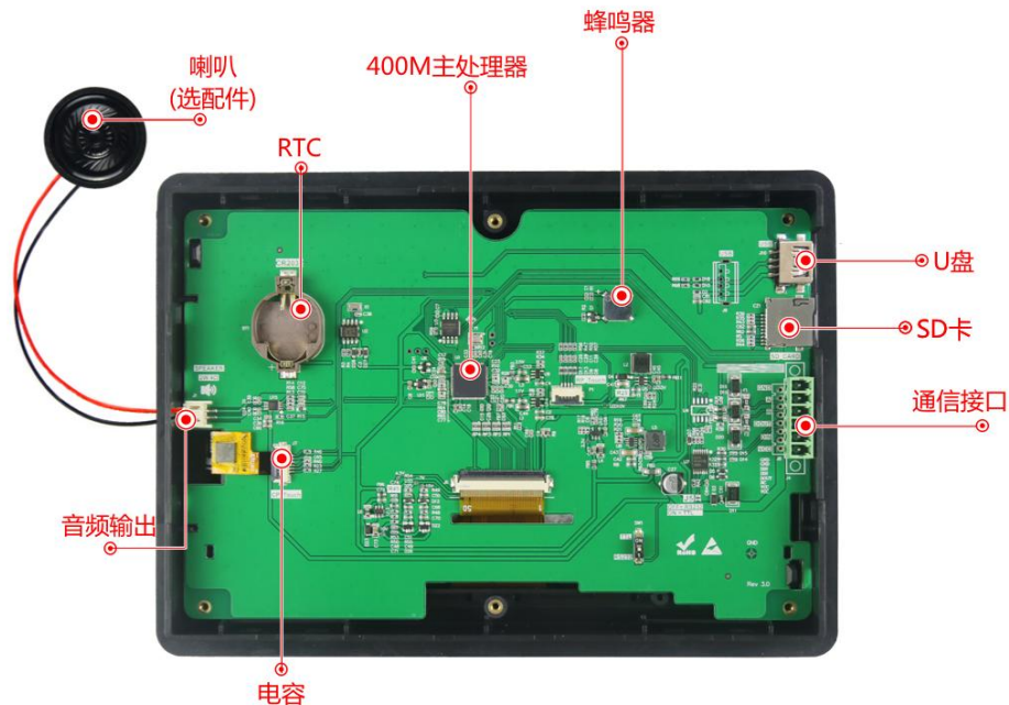
图 1-2 硬件配置图
